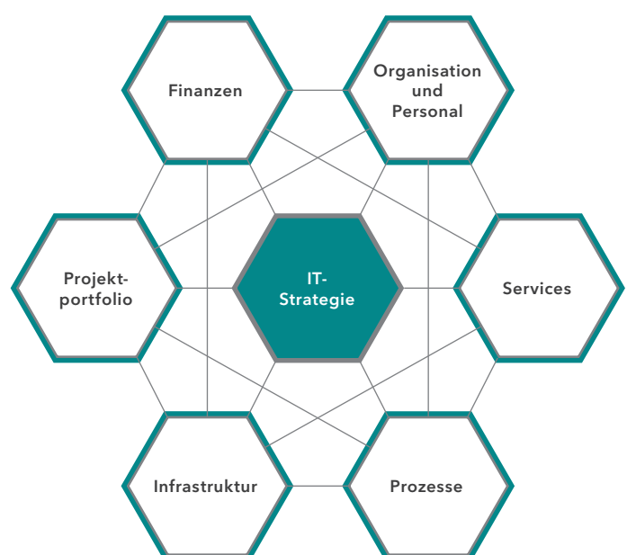
Abbildung 1 IT-Domänenmodell
